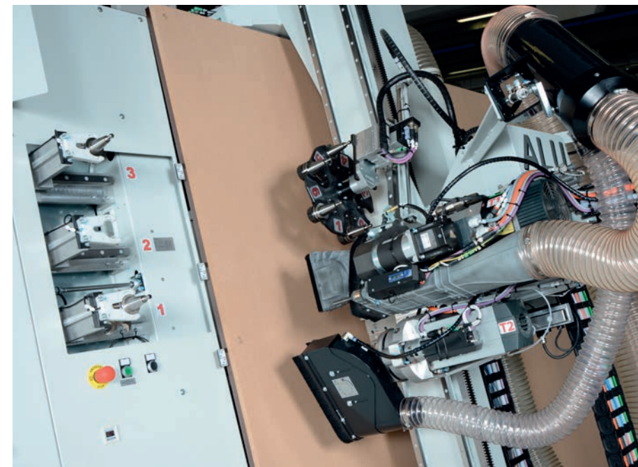
Tool changer
